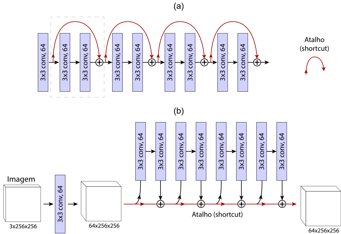
Figura 2.7: Ilustração de redes residuais. (a) Exemplo de uma rede residual composta por 4 blocos residuais. O primeiro bloco residual está indicado pelo retângulo tracejado. O bloco consiste em realizar duas convoluções (seguidas por normalização e ativação não linear). A saída das convoluções é somada com o tensor de entrada do bloco. O processo é repetido para cada bloco. (b) Uma outra forma de visualizar a mesma arquitetura de (a). Após a primeira convolução, a rede aprende o que deve ser modificado em relação à entrada para que seja obtida uma saída desejada. De forma similar, cada bloco residual aprende o que deve ser modificado em relação à entrada. Esse paradigma permite uma melhor propagação dos gradientes na rede pois existe um caminho direto entre a entrada e saída dos dados. Adicionalmente, sem qualquer treinamento a rede já possui capacidade de representar a função identidade, que apenas copia a entrada para a saída. Portanto, dizemos que cada bloco aprende o resíduo dos dados, isto é, o que deve ser mudado em relação à entrada.
