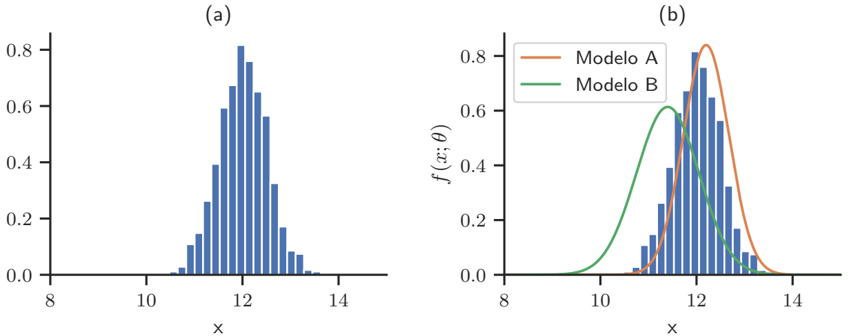
Figura 1.3: (a) Histograma de um conjunto de dados. (b) Dois possíveis modelos para a distribuição de probabilidades dos dados.
