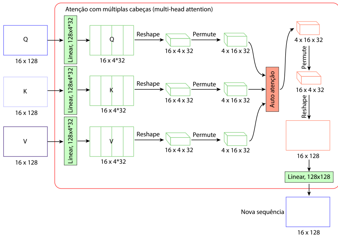
Figura 3.3: Implementação eficiente de atenção com múltiplas cabeças. Três camadas lineares são aplicadas nas entradas. Cada camada linear gera 4 * 32 = 128 novos valores para cada token. Essas camadas consistem na aplicação das 4 cabeças mostradas na Figura 3.2(b) em uma única multiplicação matricial. Uma operação de reshape é aplicada em cada resultado, gerando tensores de tamanho 16x4x32, seguida de uma operação permute, gerando tensores de tamanho 4x16x32. Essa configuração de dimensões permite aplicar a camada de auto atenção tratando a primeira dimensão (de tamanho 4) como se fosse uma dimensão de batch. O resultado é permutado e redimensionado para 16x128. Uma camada linear final é aplicada, gerando uma nova sequência de tamanho 16x128 na qual os tokens foram alterados para a inclusão de contexto.
