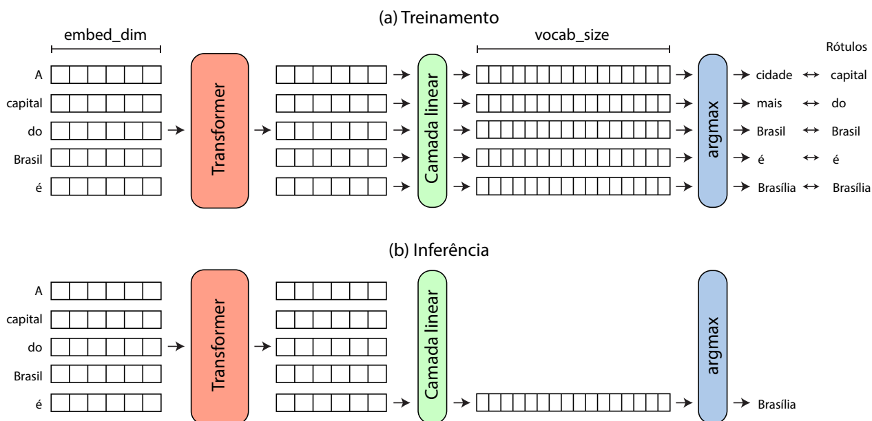
Figura 4.4: Ilustração do treinamento e inferência de um modelo de texto generativo. (a) Cada token de uma sentença de entrada é transformado em um vetor de valores através de uma camada de embedding. O tamanho do vetor é usualmente chamado de embed_dim ou model_dim . Um transformer processa os dados e gera novos vetores de mesmo tamanho, mas com significado semântico enriquecido. Uma camada linear é utilizada para gerar scores para cada um dos possíveis tokens do vocabulário do modelo. Modelos de língua inglesa em geral possuem vocab_size \approx 40000 . Modelos multilinguagem como o Llama podem possuir até vocab_size \approx 128000 . O token de maior score para cada posição i é selecionado e comparado com o token na posição i+1 da sentença de entrada. A comparação é feita através da entropia cruzada. (b) No momento da inferência, um processo similar é repetido, mas a camada linear é aplicada apenas no vetor associado ao último token.
